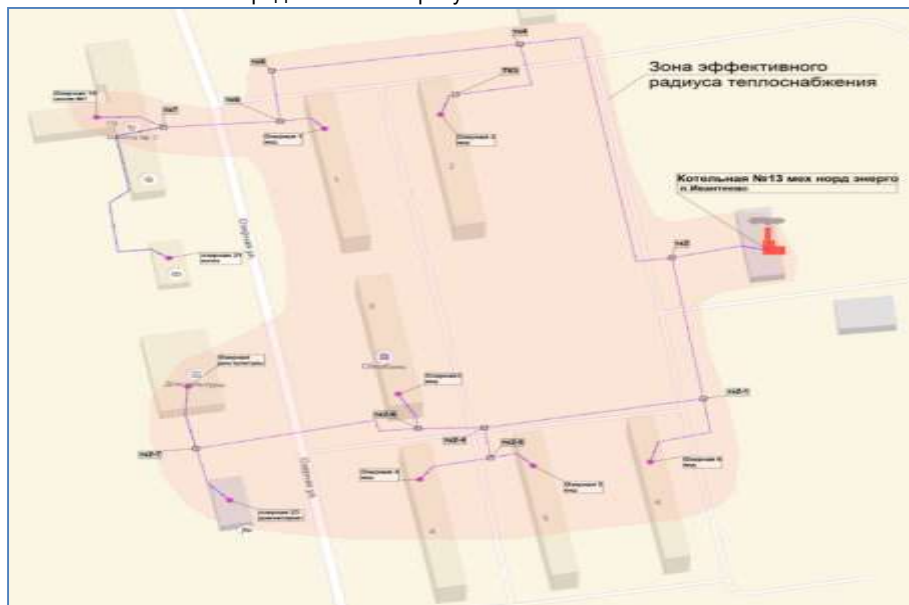
Рисунок 2. Зона эффективного радиуса теплоснабжения котельной № 13
