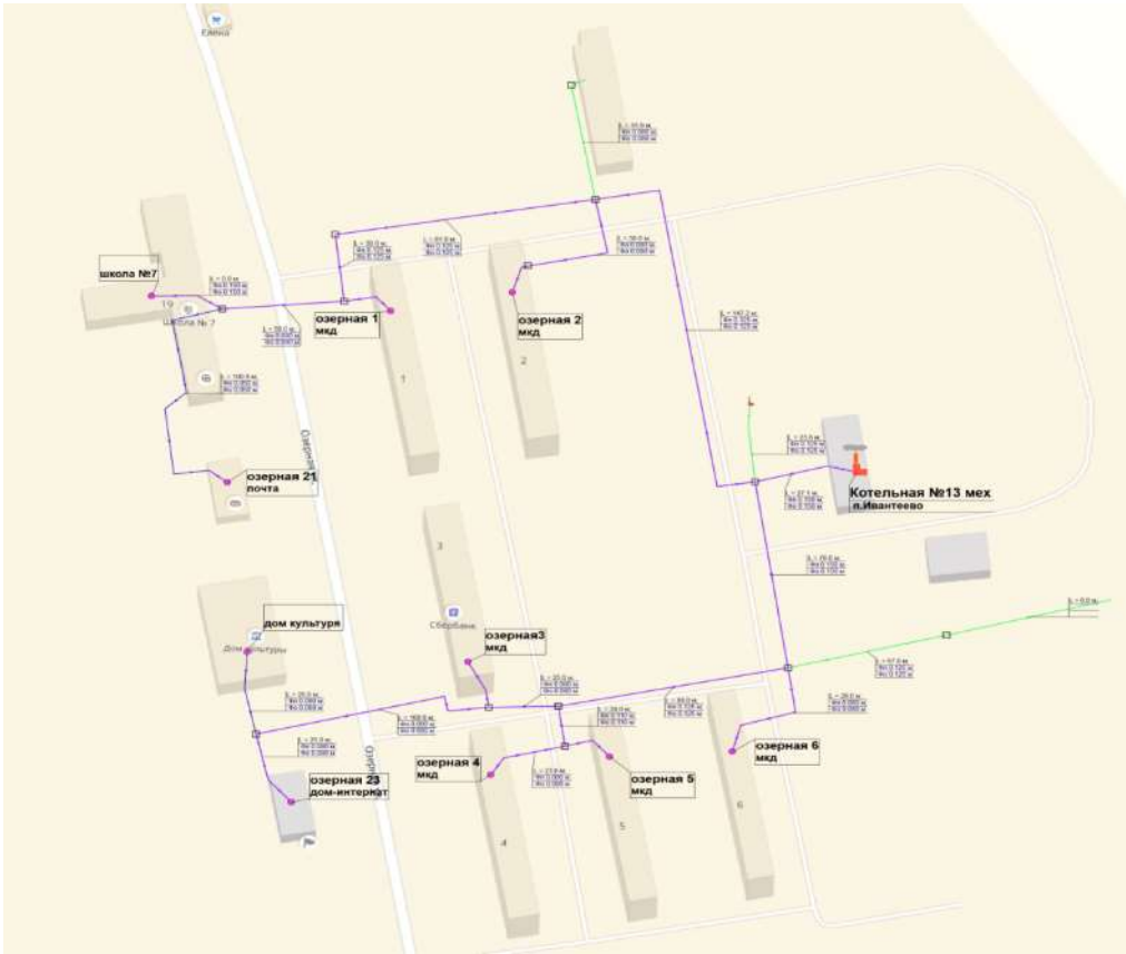
Рисунок 1. Схема тепловых сетей котельной № 13 д. Ивантеево
