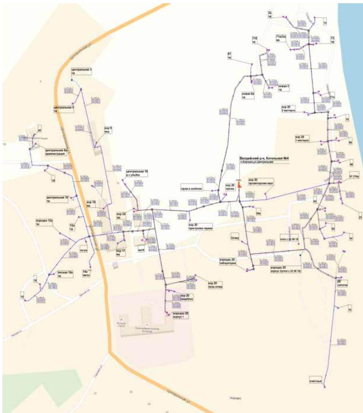
Рисунок 1. Схема тепловых сетей котельной № 4 п. Короцко, ул. Озерная
