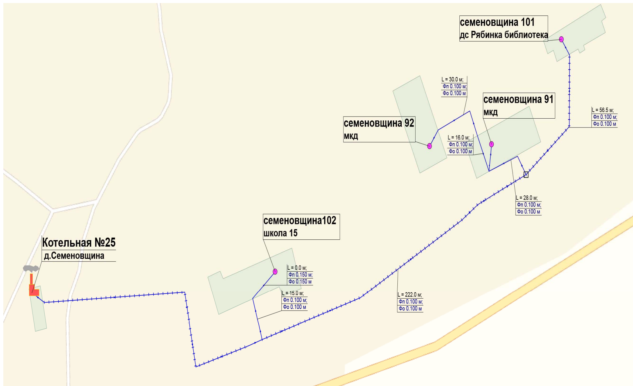
Рисунок 1. Схема тепловых сетей котельной № 25, д. Семеновщина
