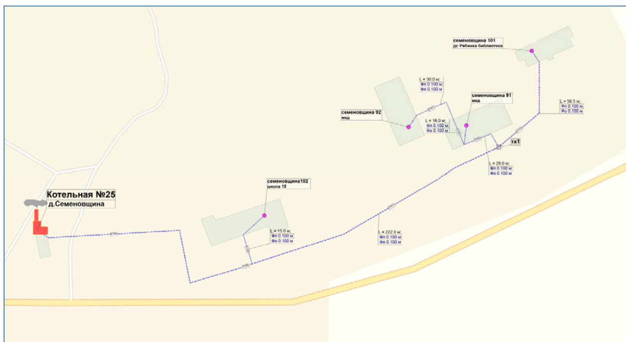
Рисунок 1. Схема тепловых сетей котельной № 25
