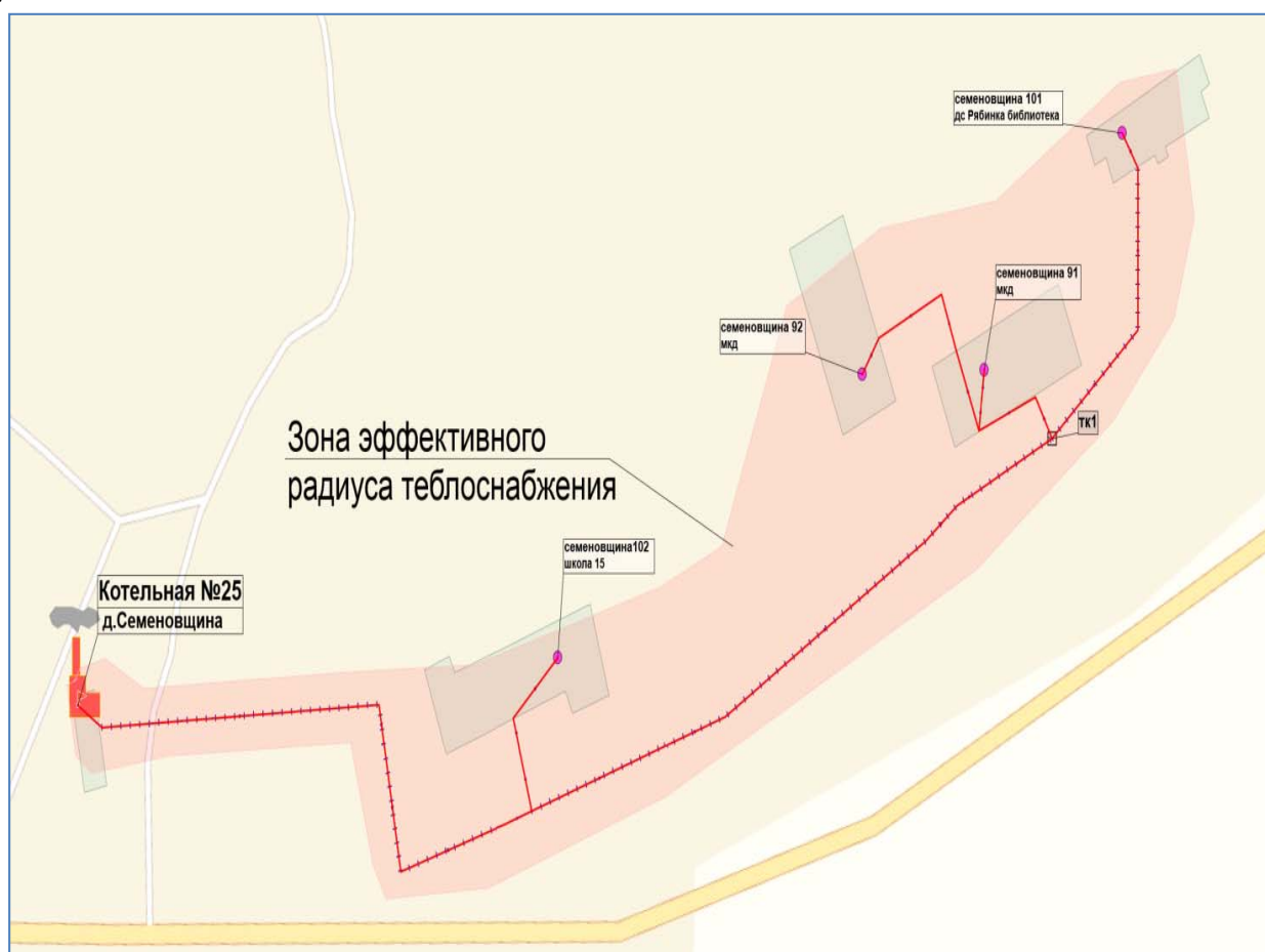
Рисунок 2. Зона эффективного радиуса теплоснабжения котельной №25
