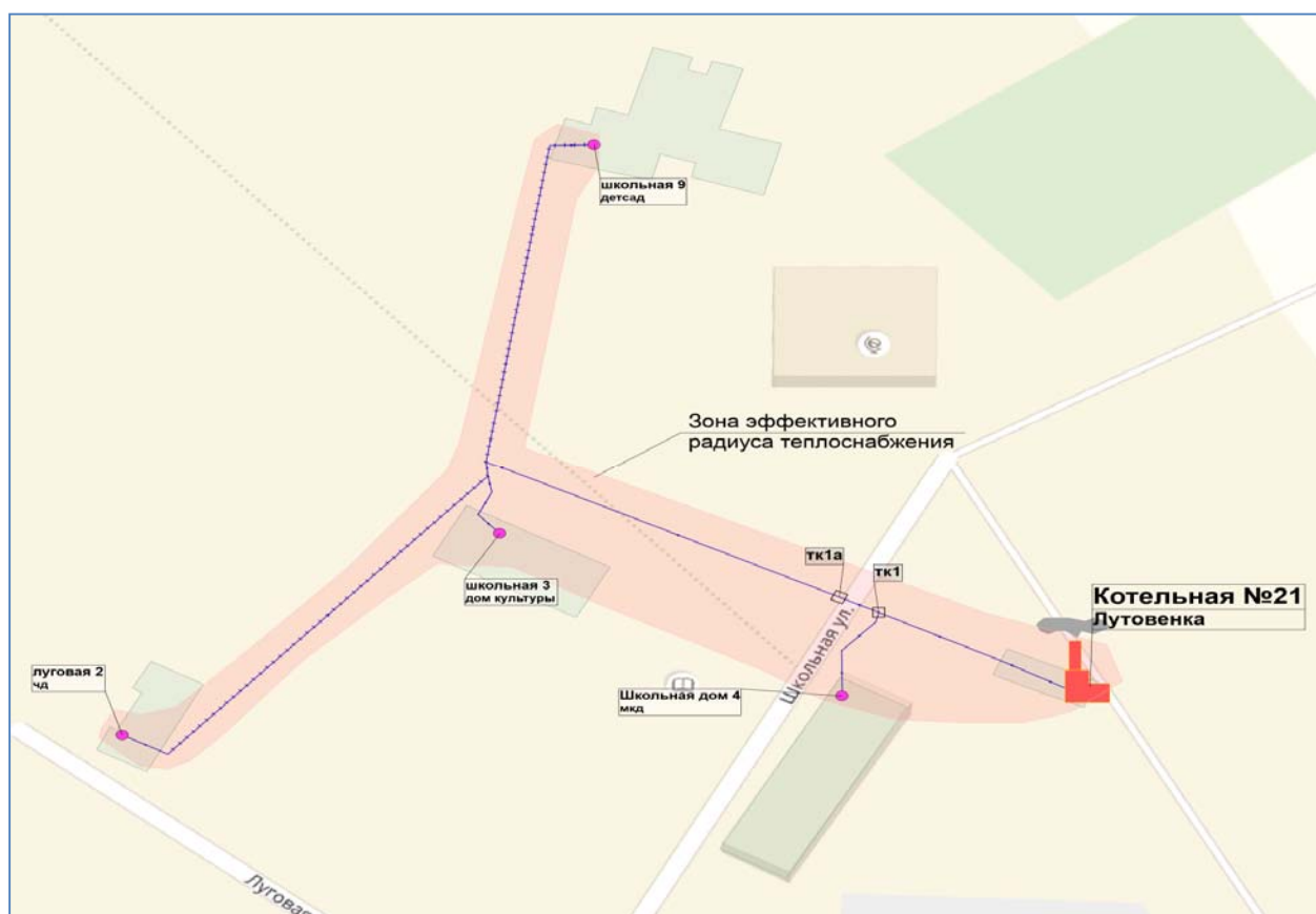
Рисунок 3. Зона эффективного радиуса теплоснабжения котельной №21
