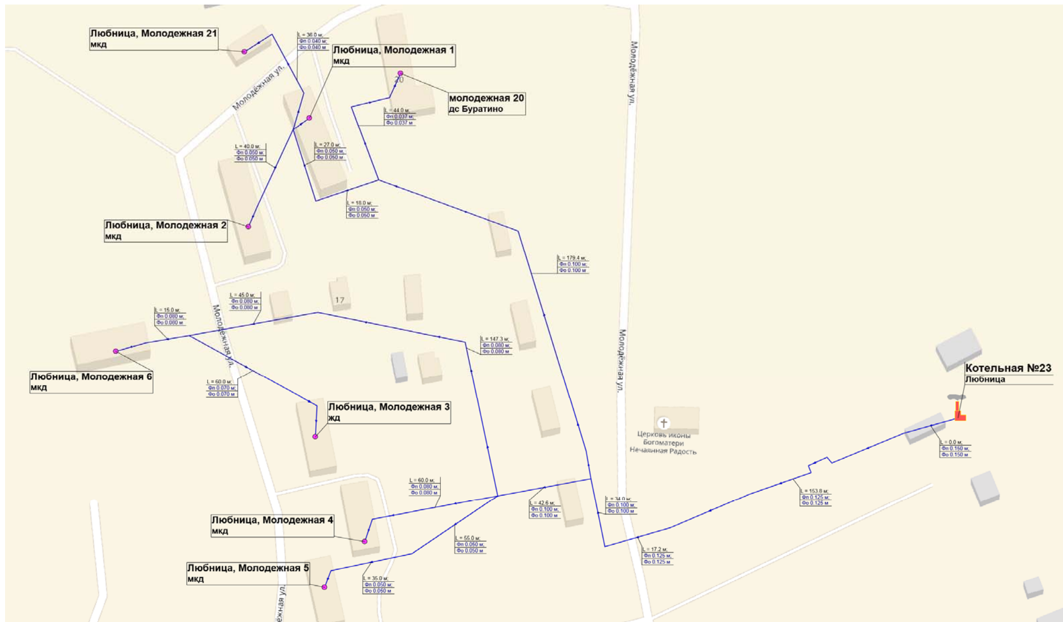
Рисунок 2. Схема тепловых сетей котельной № 23 д. Любница.
